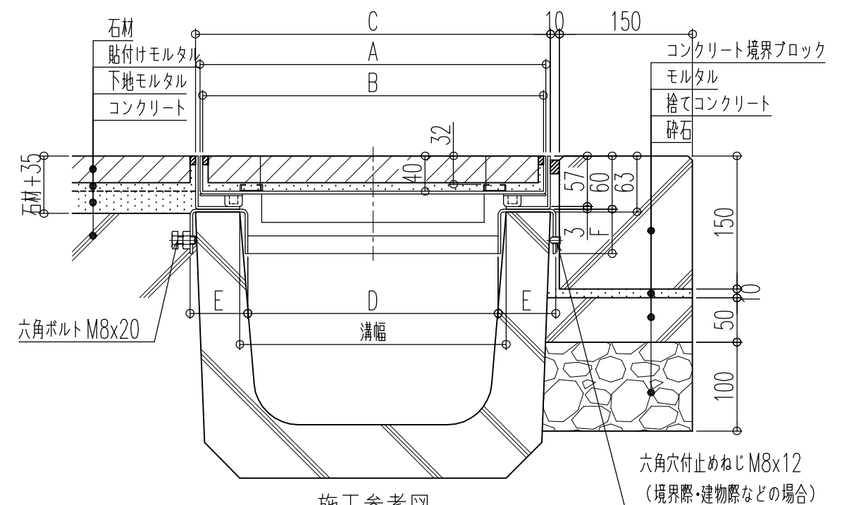
施工参考図
